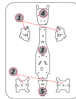
HONDA Rincon 680
